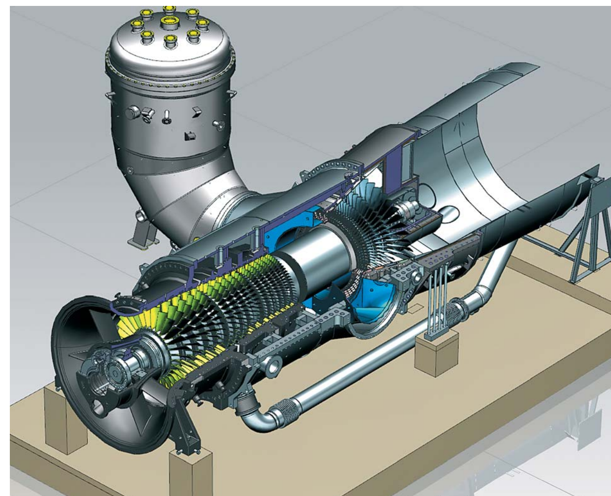
ГАЗОВАЯ ТУРБИНА
