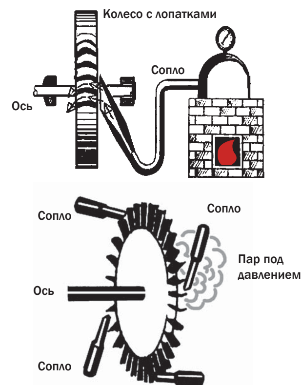
Паровая турбина Лавала
