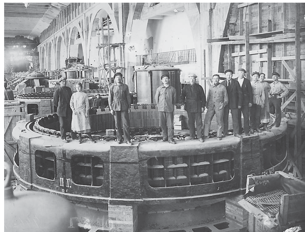
Статор генератора Волховской ГЭС. 1926 год
