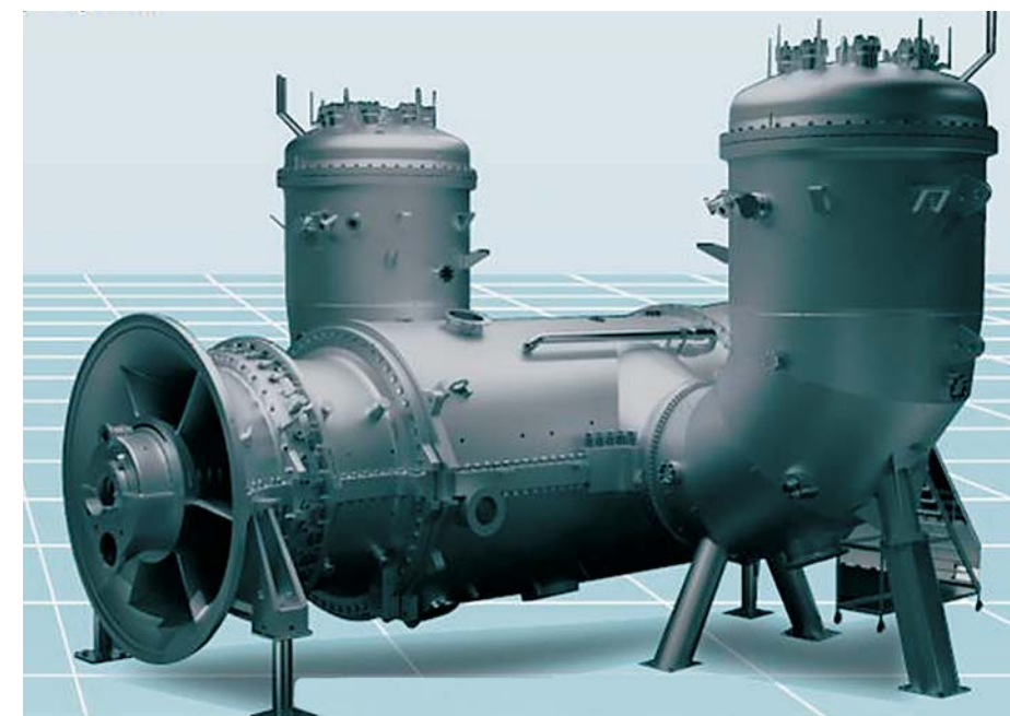
ГАЗОВАЯ ТУРБИНА
