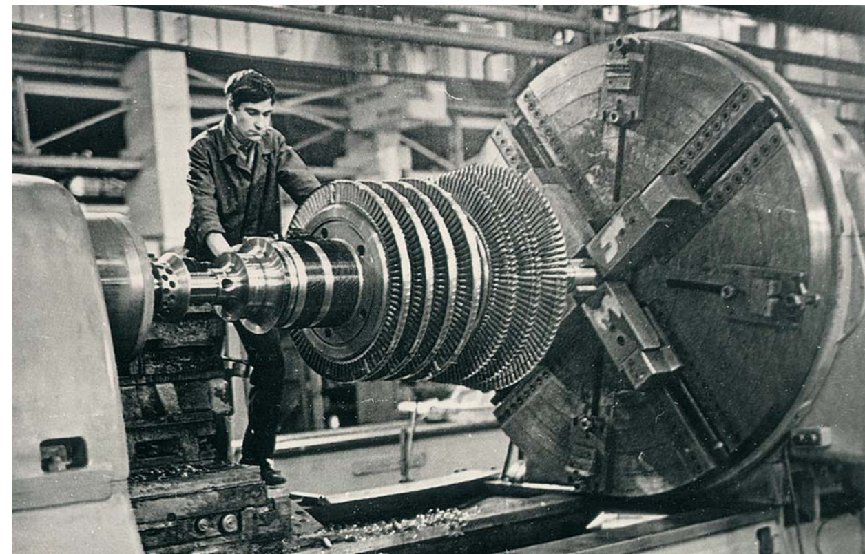
Обработка ротора турбины. 1960 год
